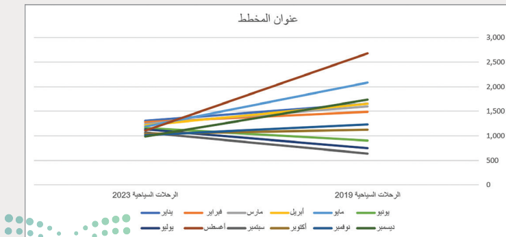
شكل 4.22: مخطط خطي غير مفهوم
