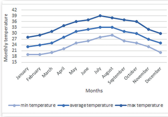
الشكل 3.37: مخطط خطي يوضح المتوسط السنوي لدرجات الحرارة المنخفضة والمتوسطة المسجلة في آنّها
