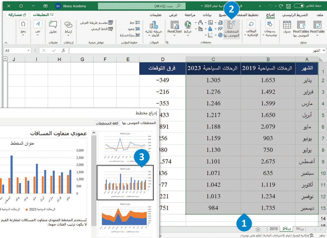
شكل 4.20: إنشاء مخطط عمودي متفاوت المسافات
