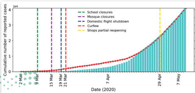
شكل 4.1: تقييم النموذج التنبؤي مع العدد الفعلي والعدد المتوقع لحالات الإصابة (الشكلية يومياً)
