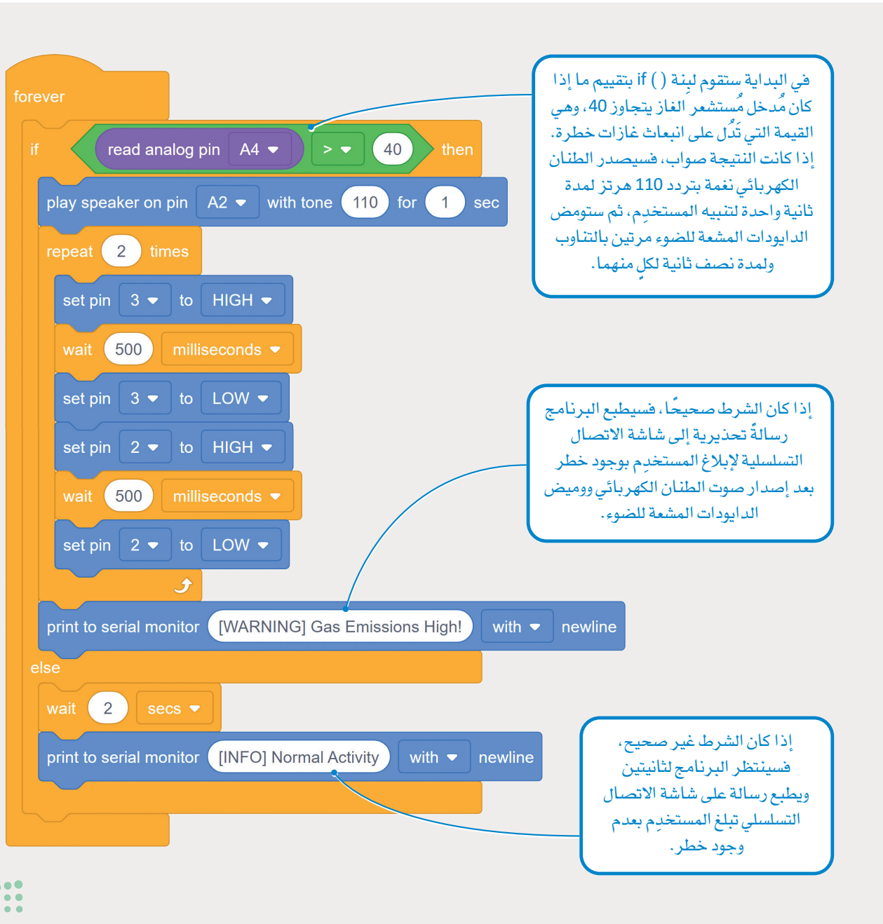
شكل 3.40: برنامج نظام إنذار تسرب الغاز
