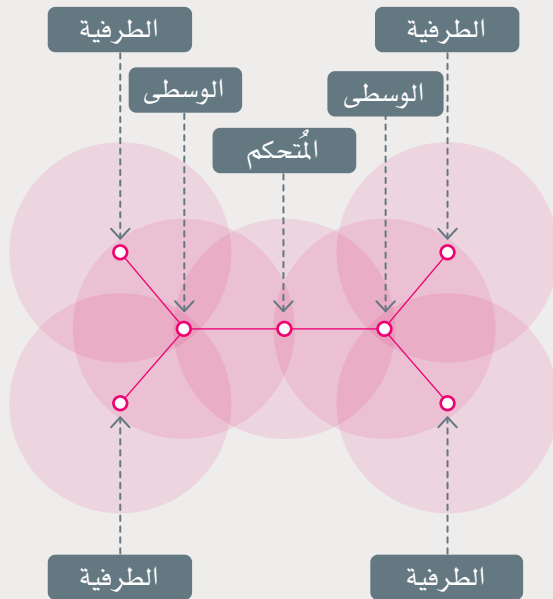
شكل 8.12: العقد ووظائفها
