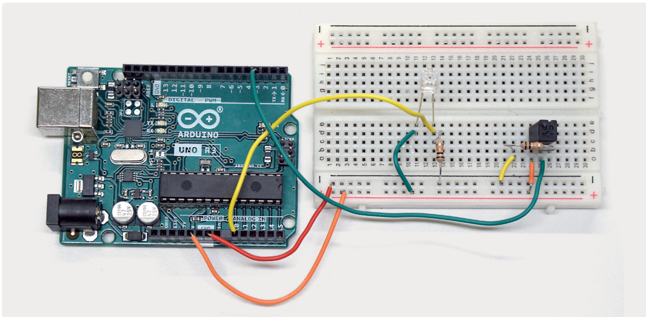
شكل 7.17: صورة للدائرة
