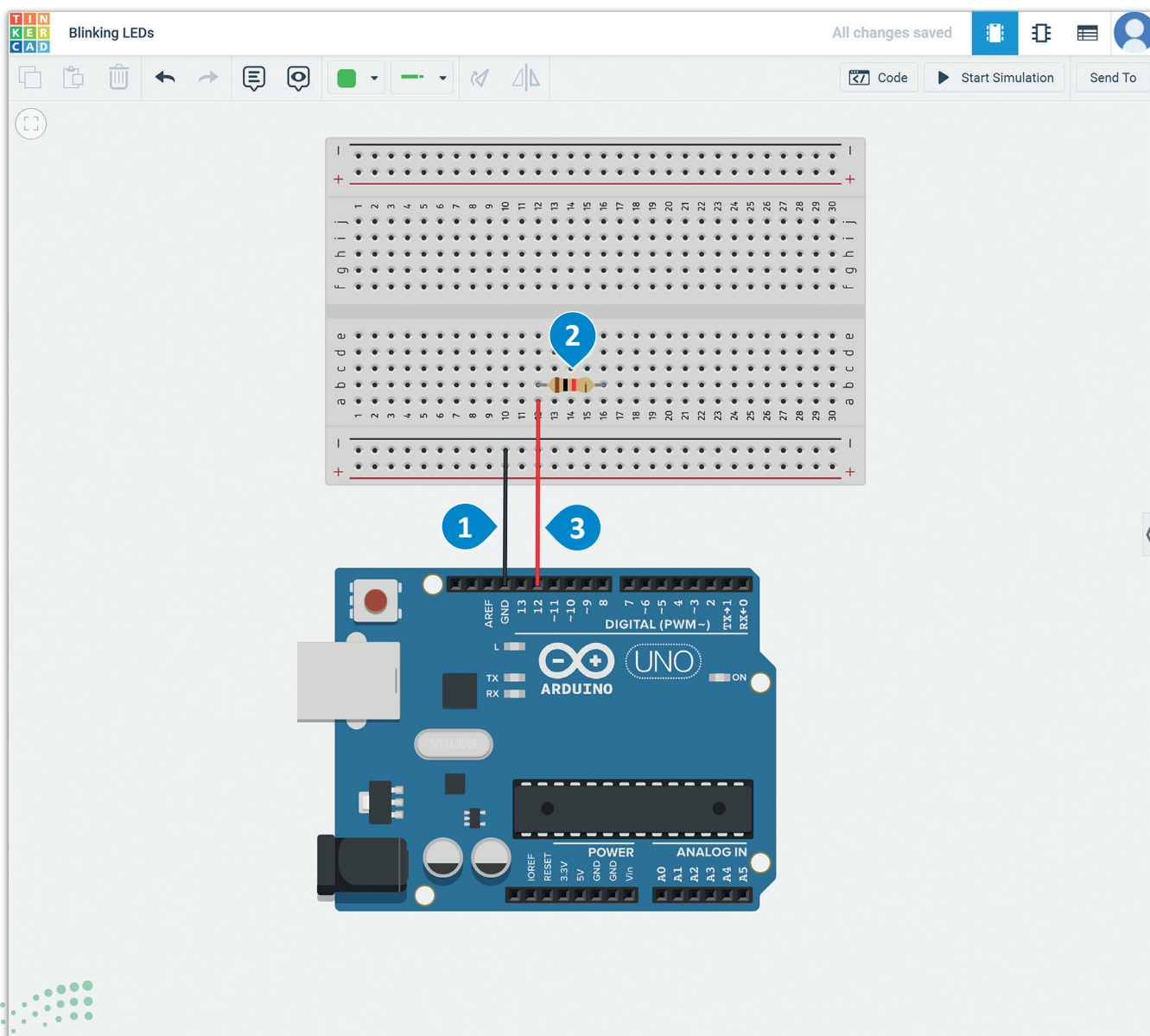
شكل 4.10: توصيل الأردوينو
