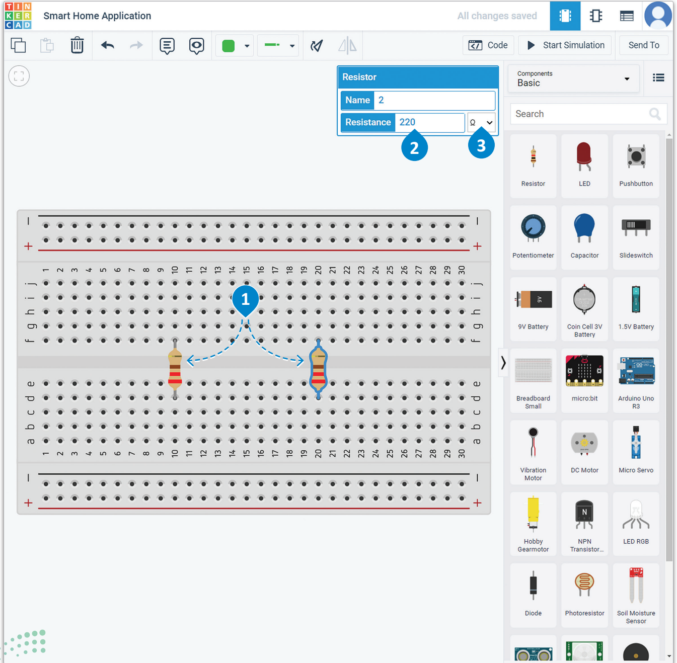
شكل 3.11: إضافة المقاومات إلى لوحة توصيل الدوائر
