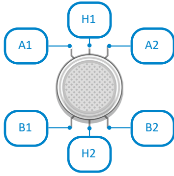
شكل 3.31: مُستشعر الغاز
