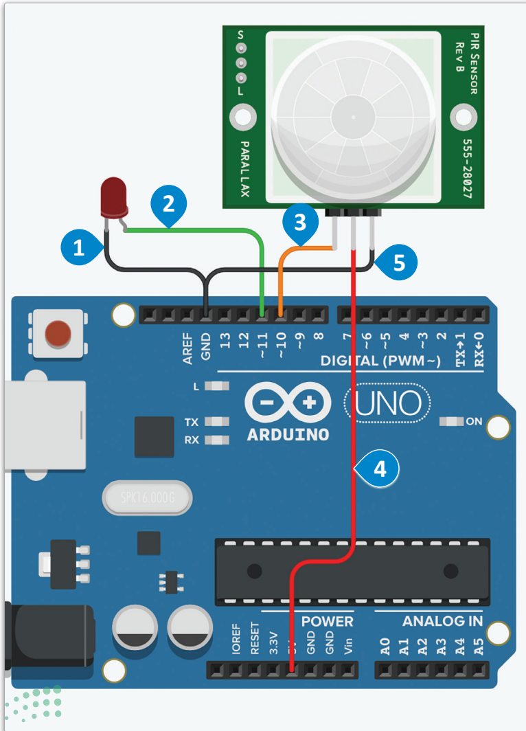
شكل 6.14: توصيل الدائرة
