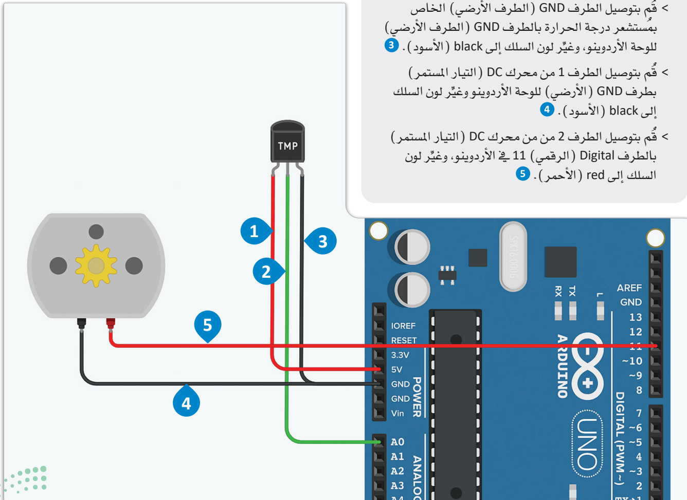
شكل 6.16: توصيل الدائرة
