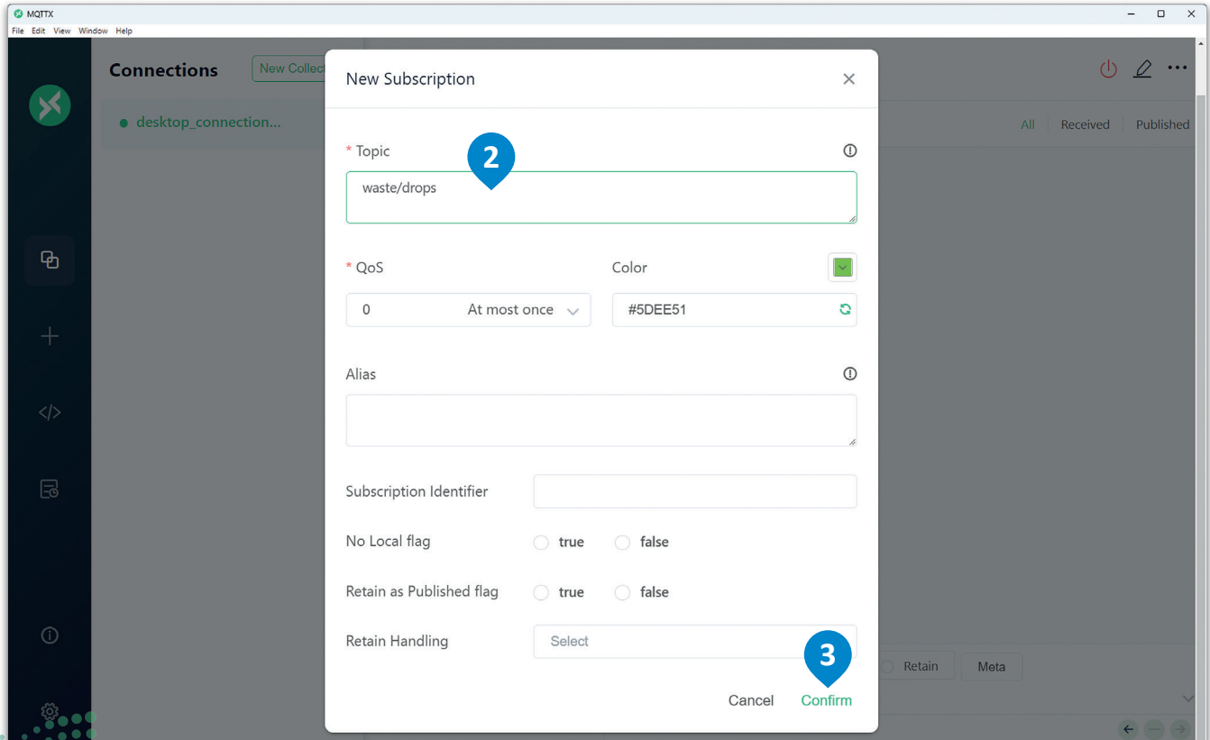
شكل 7.19: استخدام MQTTX للاشتراك في موضوع محدد
