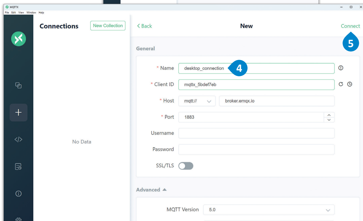
شكل 7.12: تكوين الاتصال بوسيط EMQX مع MQTTX
