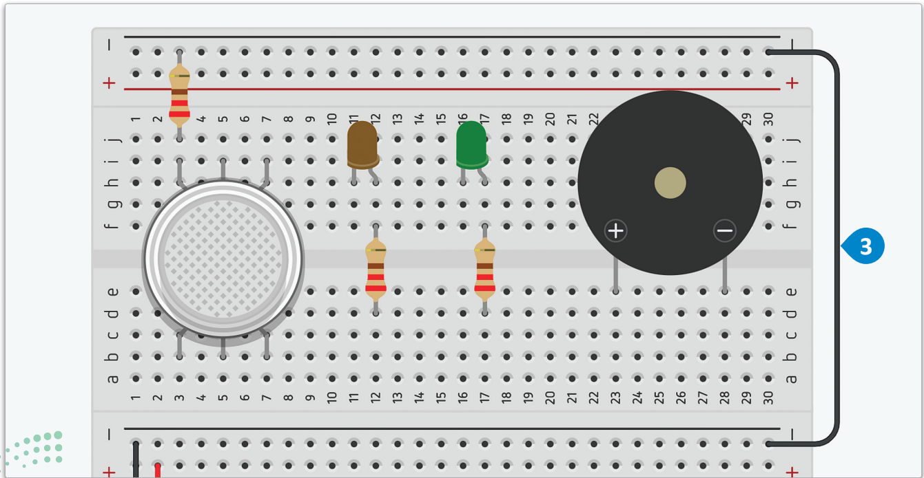
شكل 3.35: توصيل جهاز تحكم الأردوينو الدقيق
