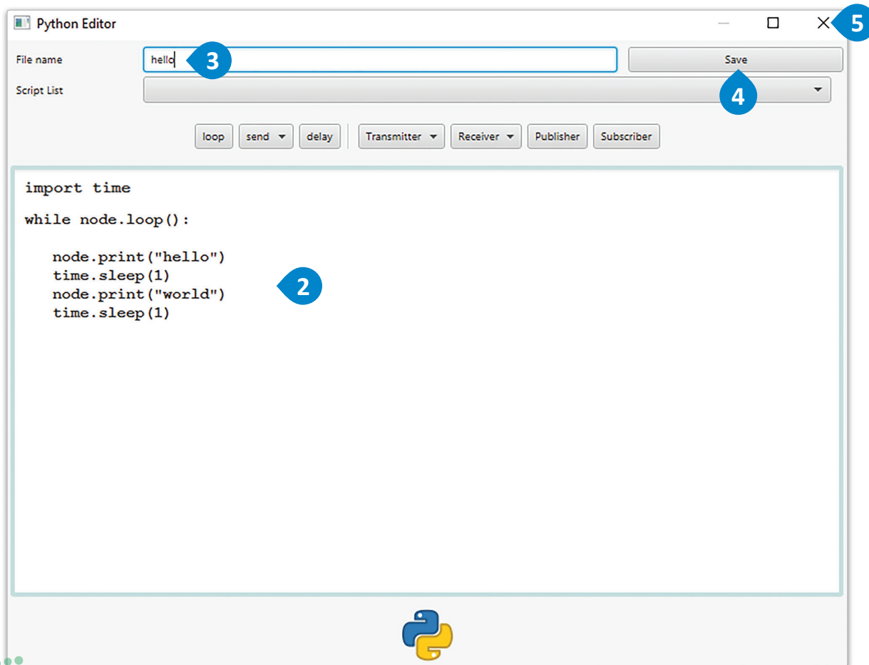
شكل 8.9: مُحرر البايثون
