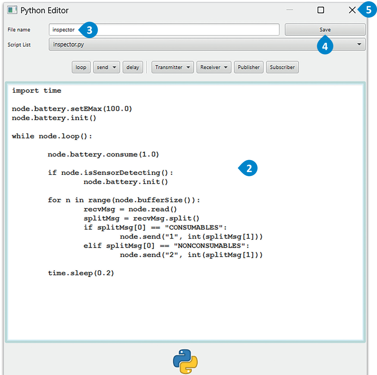
شكل 8.26: إنشاء المقطع البرمجي
