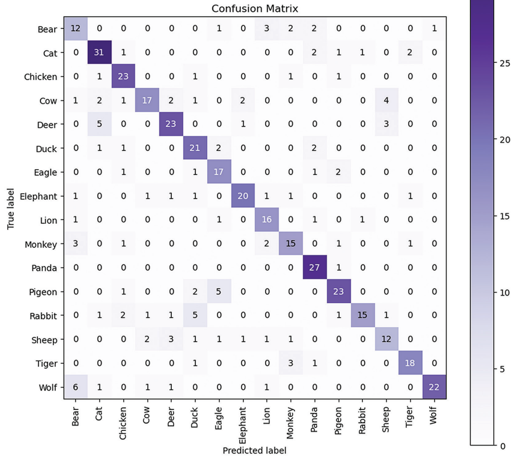
شكل 4.11: مصفوفة الدقة لأداء خوارزمية SGDClassifier
