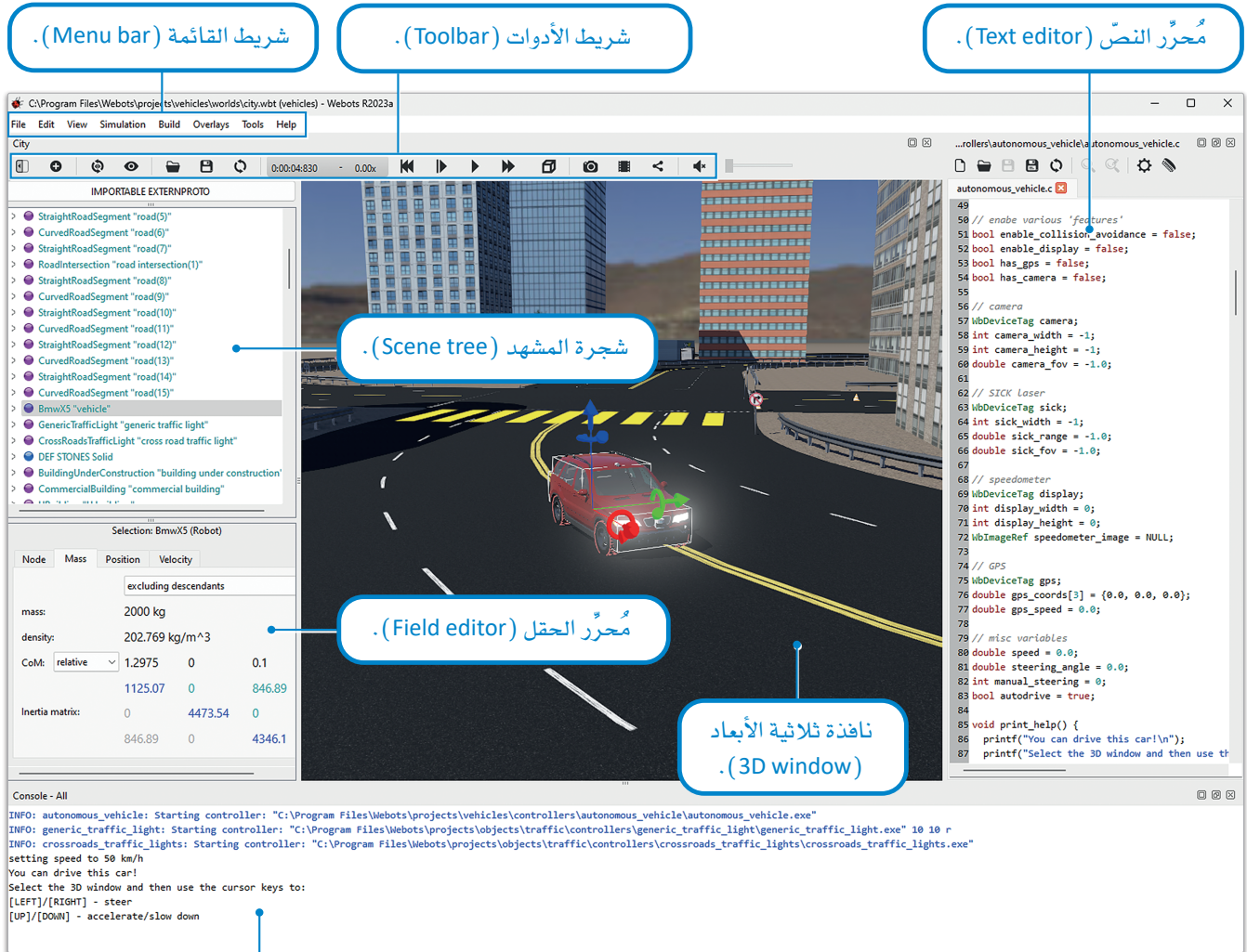
شكل 6.7: نافذة ويبوتس
