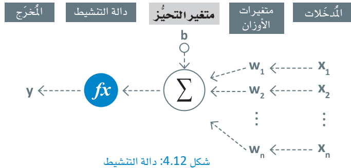
شكل 4.12: دالة التنشيط
