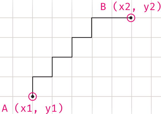
شكل 2.25: مسافة مانهاتن
