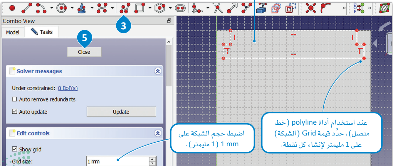
شكل 3.47: إنشاء رسم تخطيطي على السطح العلوي
