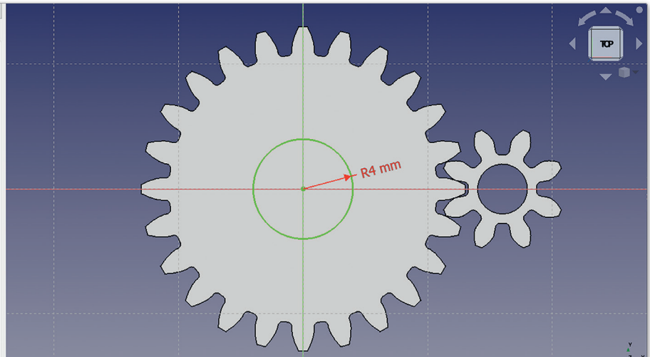
شكل 2.56: إنشاء دائرة
