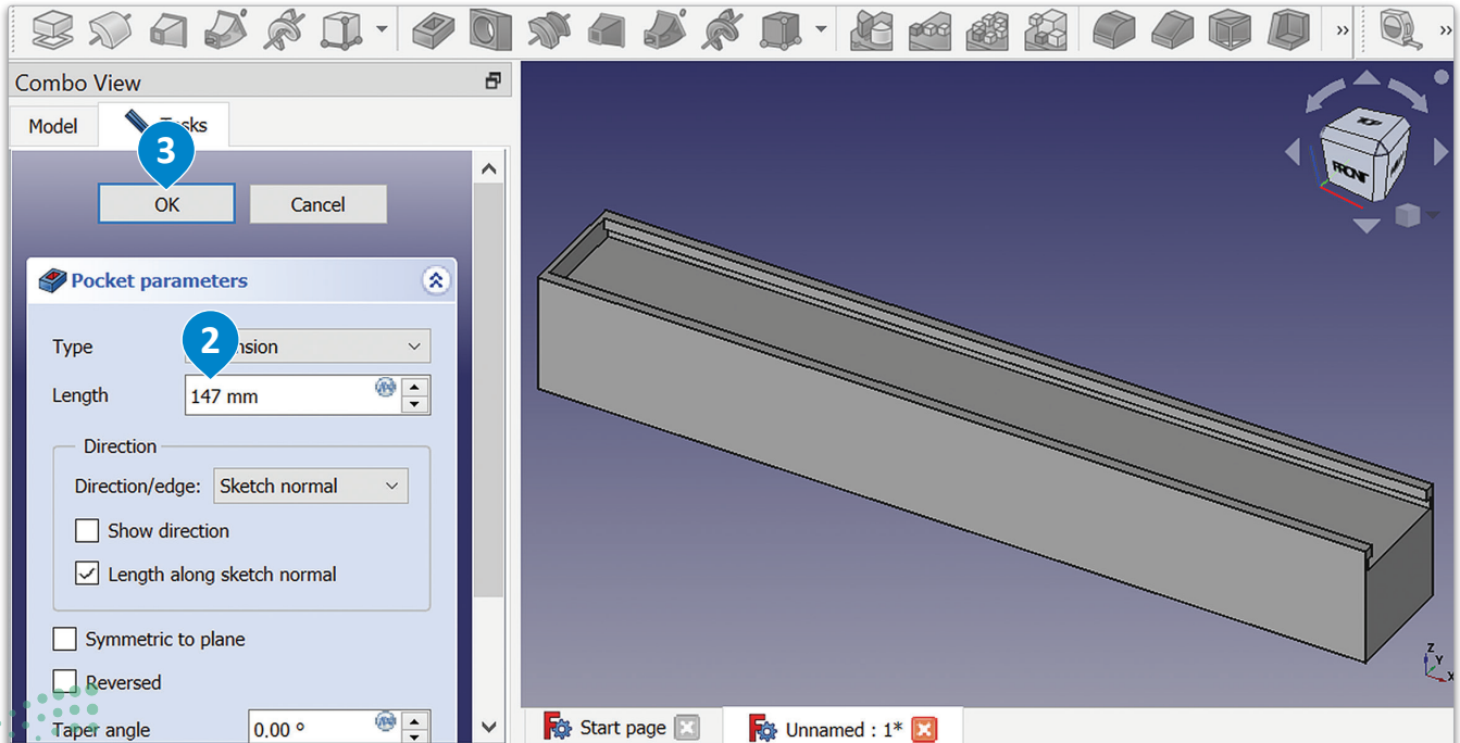
شكل 3.48: إنشاء التجويف
