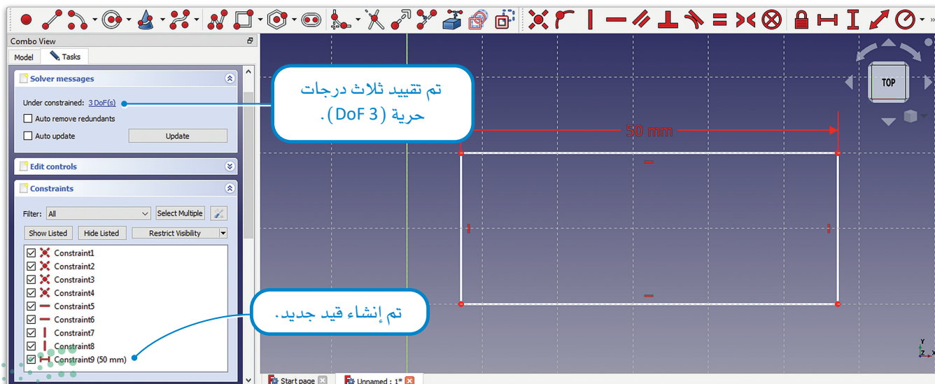
شكل 2.34: تقييد المسافة الأفقية
