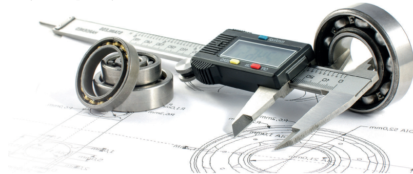
شكل 1.8: استخدام المسمك الإلكتروني للقياسات الدقيقة
