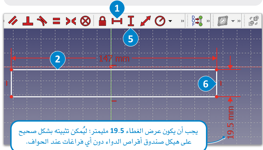
شكل 3.60: تقييد المسافة الأفقية والرأسية
