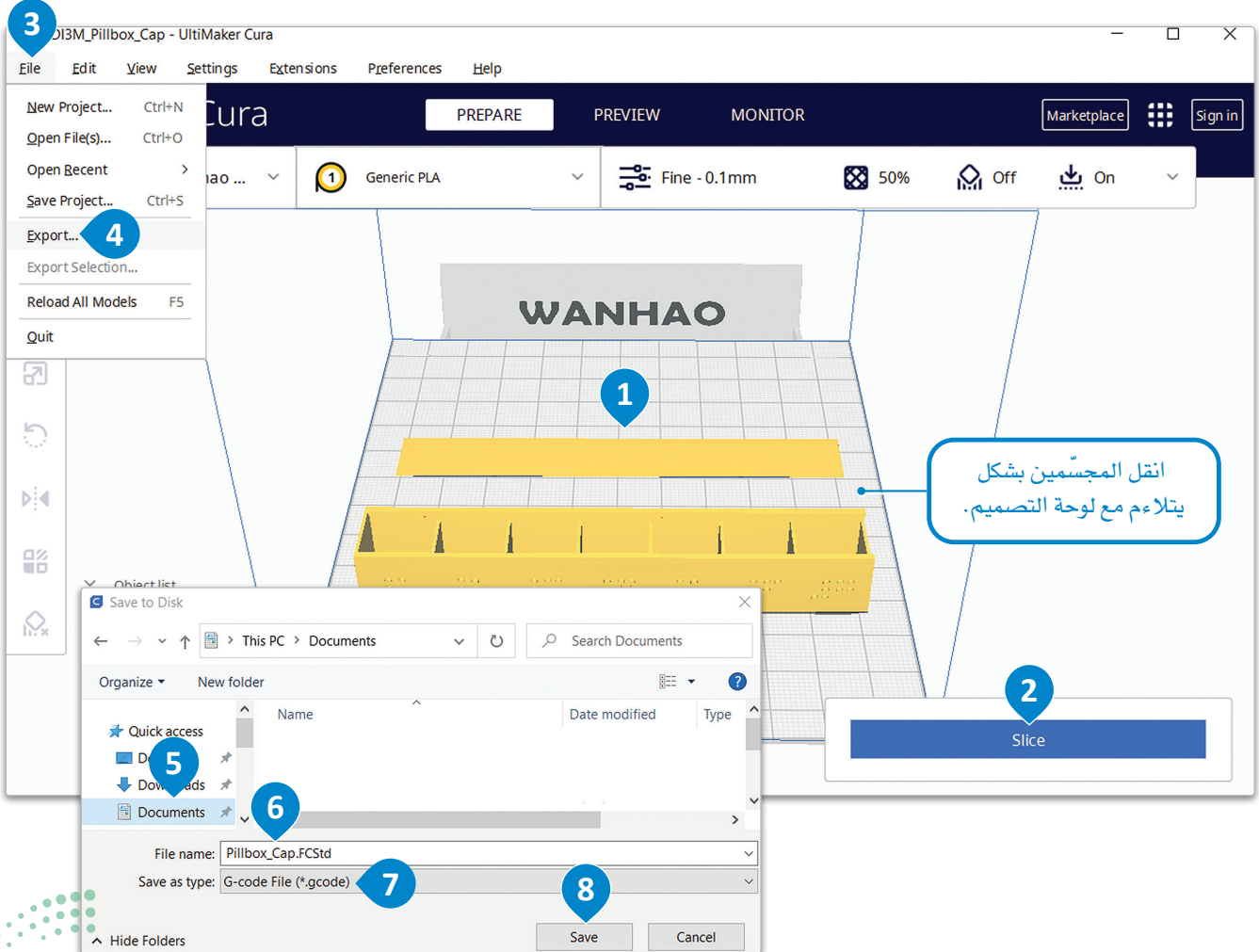
شكل 3.62: تصدير النموذجين
