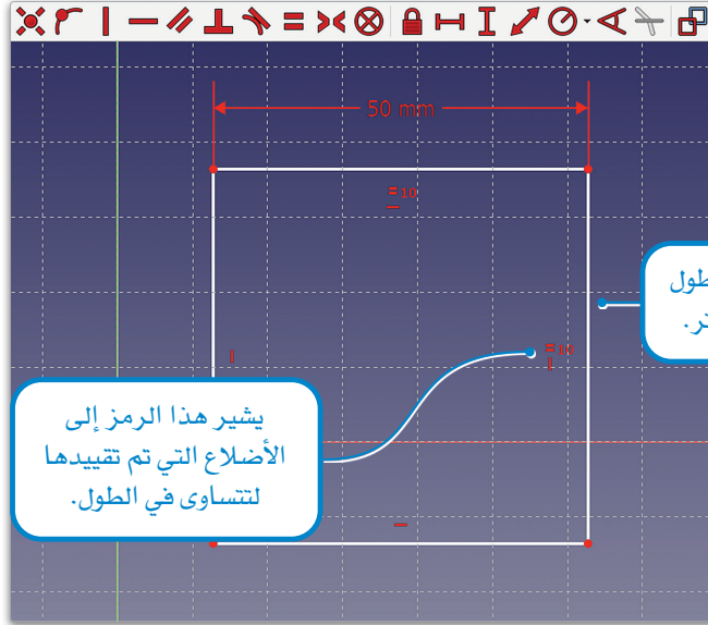
شكل 2.35: جعل الأضلاع متساوية
