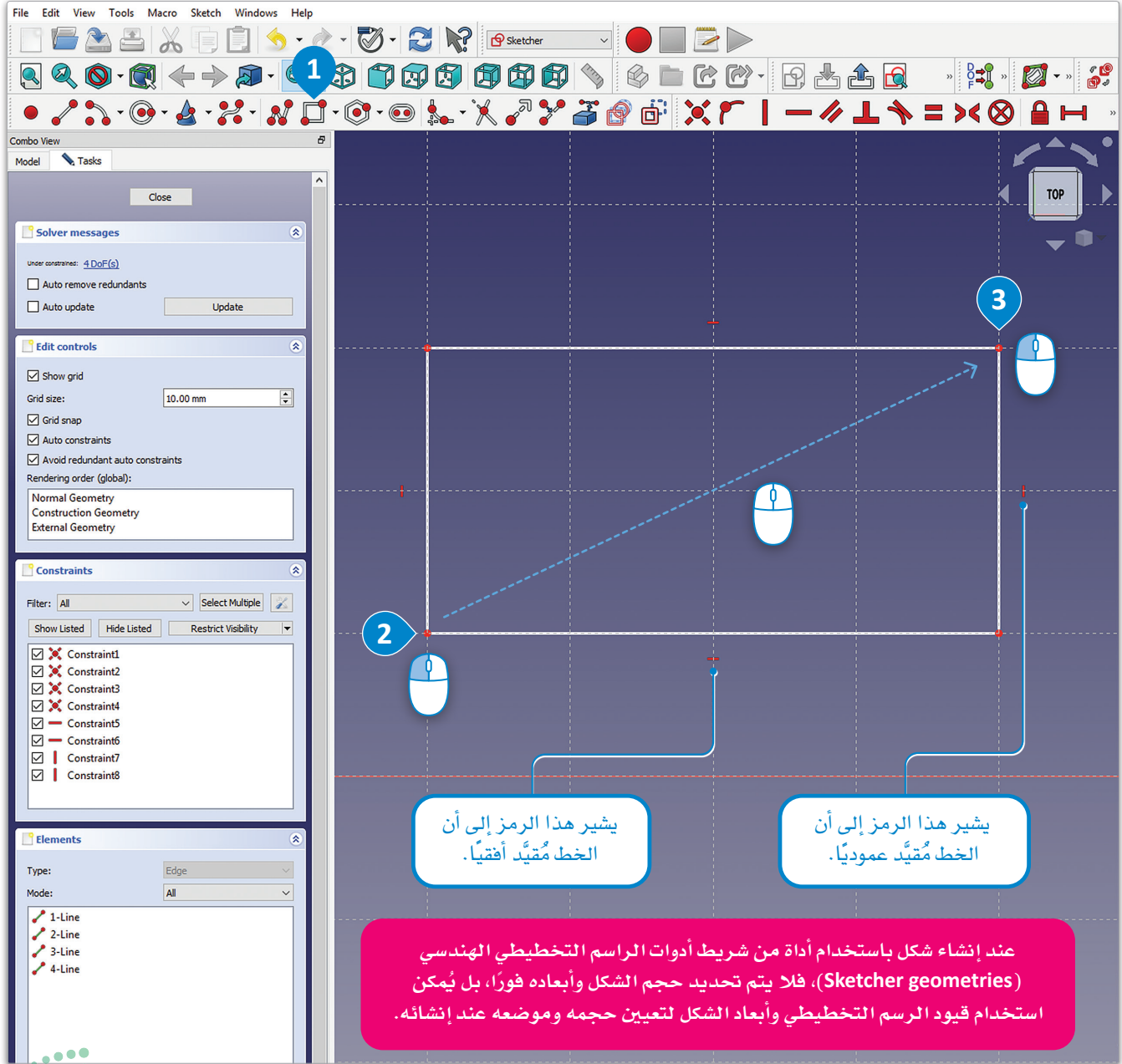
شكل 2.33: إنشاء مستطيل
