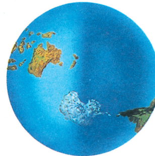
نصف الكرة المحيطي
