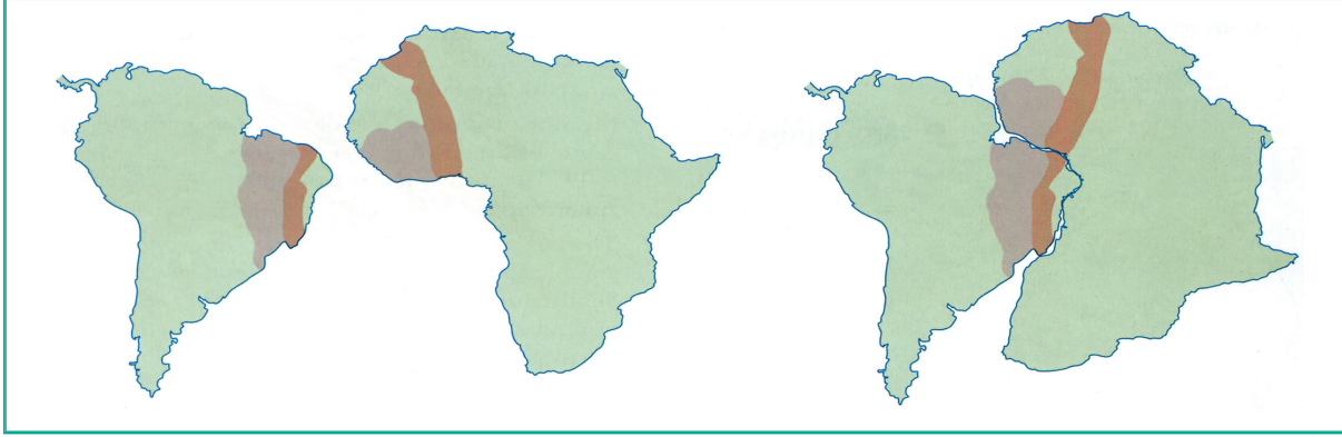
يُلحَظ التشابه بين الساحل الغربي لإفريقيا والساحل الشرقي لأمريكا الجنوبية.
