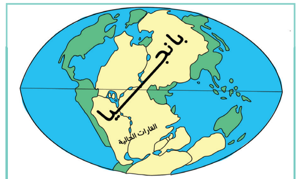
بانجيا (أم القارات)
