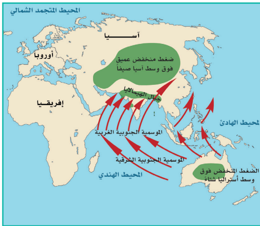
الرياح الموسمية الصيفية
